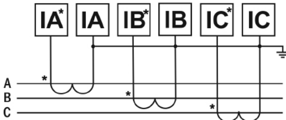
Рис. 6– Подключение трансформатора тока
