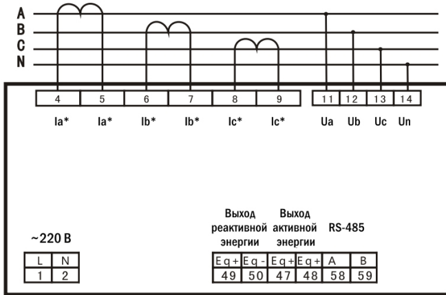
Рис. 3– Клеммы подключения
